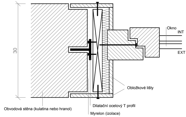
Varianta B (srub i roubenka)
