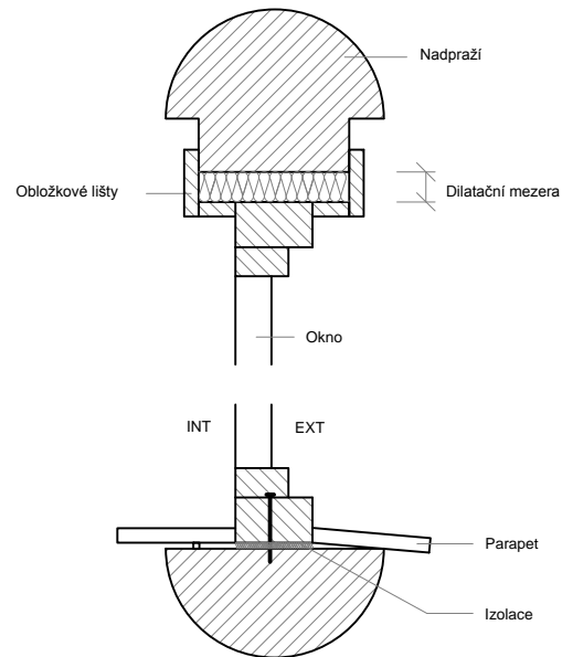
Varianta B (srub i roubenka)
